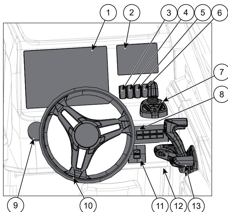
Figur 5.1 Yamarin 63 DC/BR styrestasjonskontroller
