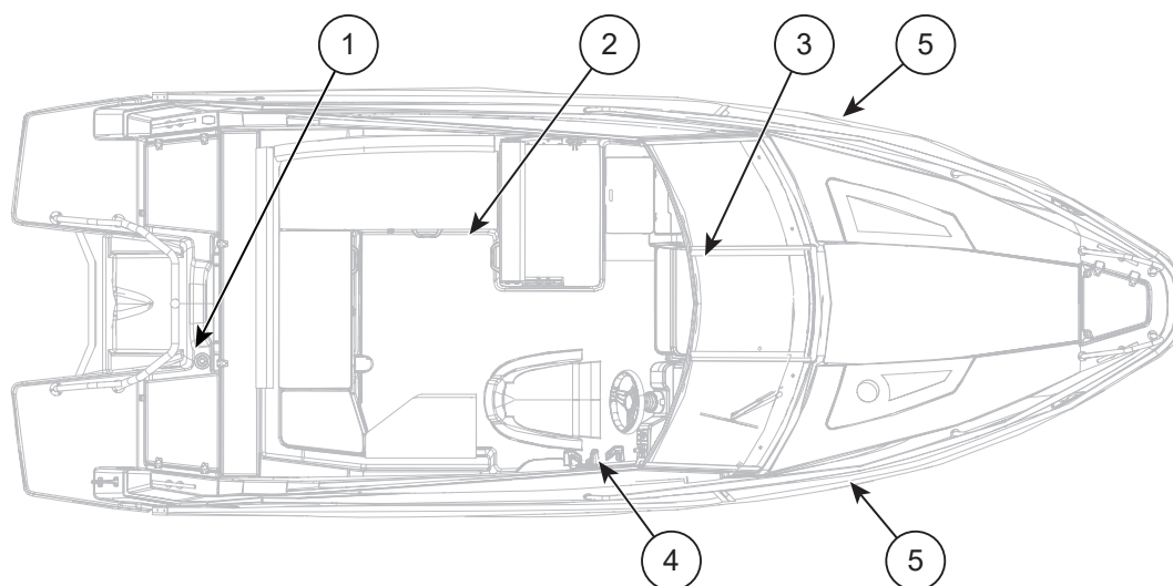
Figur 2.1 Yamarin 63 DC sikkerhetsmerker.
