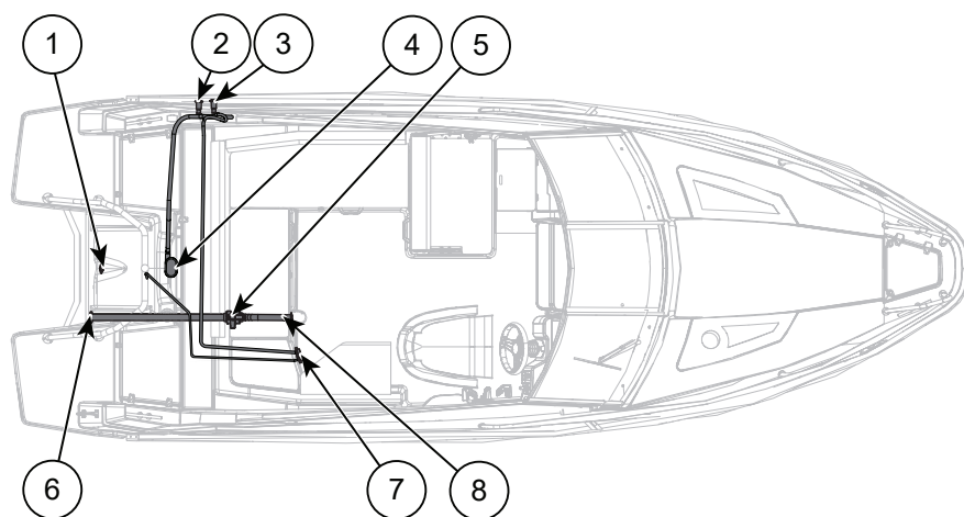
Figur 9.1 Yamarin 63 DC lensepumper og drenering
